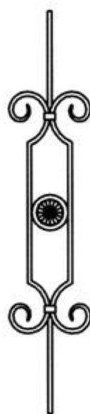
EIW 142 □16 x 8mm SCROLLS : Ø65 ROSETTE 600 x 200 H HEB / PL
