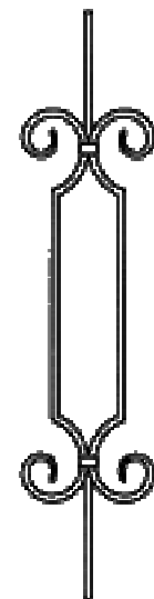
EIW 209 □16 x 8mm SCROLLS : 16 x 8mm 600 H x 200 W HEB / PL
