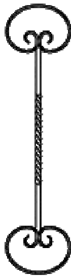
EIW 202 □16mm SCROLL : 16 x 8mm 900 H x 216 W HEB / TBS / PL
