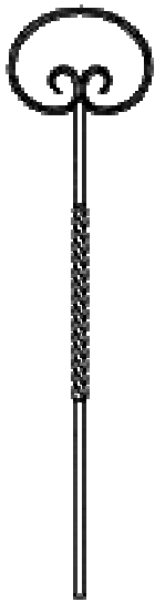
EIW 200 □16mm SCROLL : 16 x 8mm 900 H x 216 W HEB / TBS / PL
