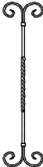
EIW 206 □16mm SCROLLS : 16 x 8mm 900 H x 216 W HEB / TBS / PL
