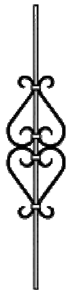
EIW 119 □ 12 / Ø14mm SCROLLS : 13 x 6mm 500 H x 202 W HEB / PL
