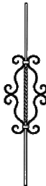
EIW 123 □12-16 / Ø14mm SCROLLS : 13 x 6 / 16 x 8 430 H x 230 W HEB / TBS / PL
